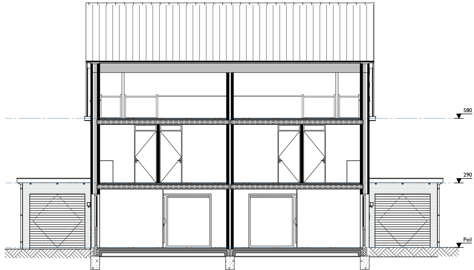
Doorsnede A-A
