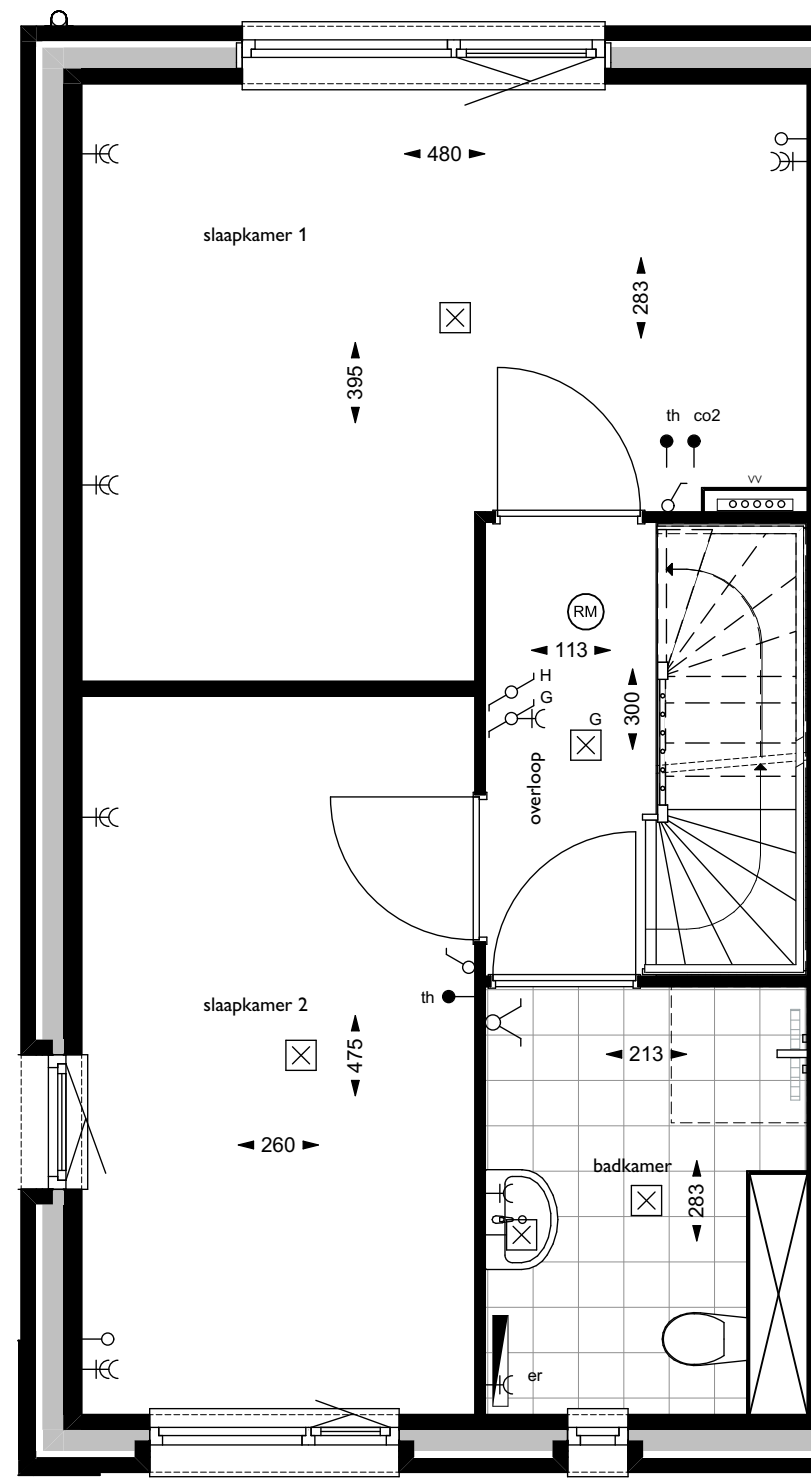
bouwnummer 43 eerste verdieping
