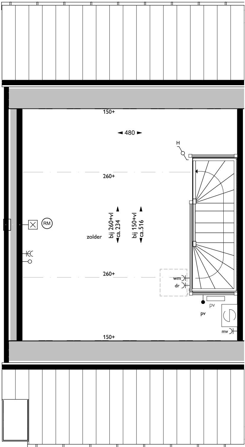
bouwnummer 43 tweede verdieping
