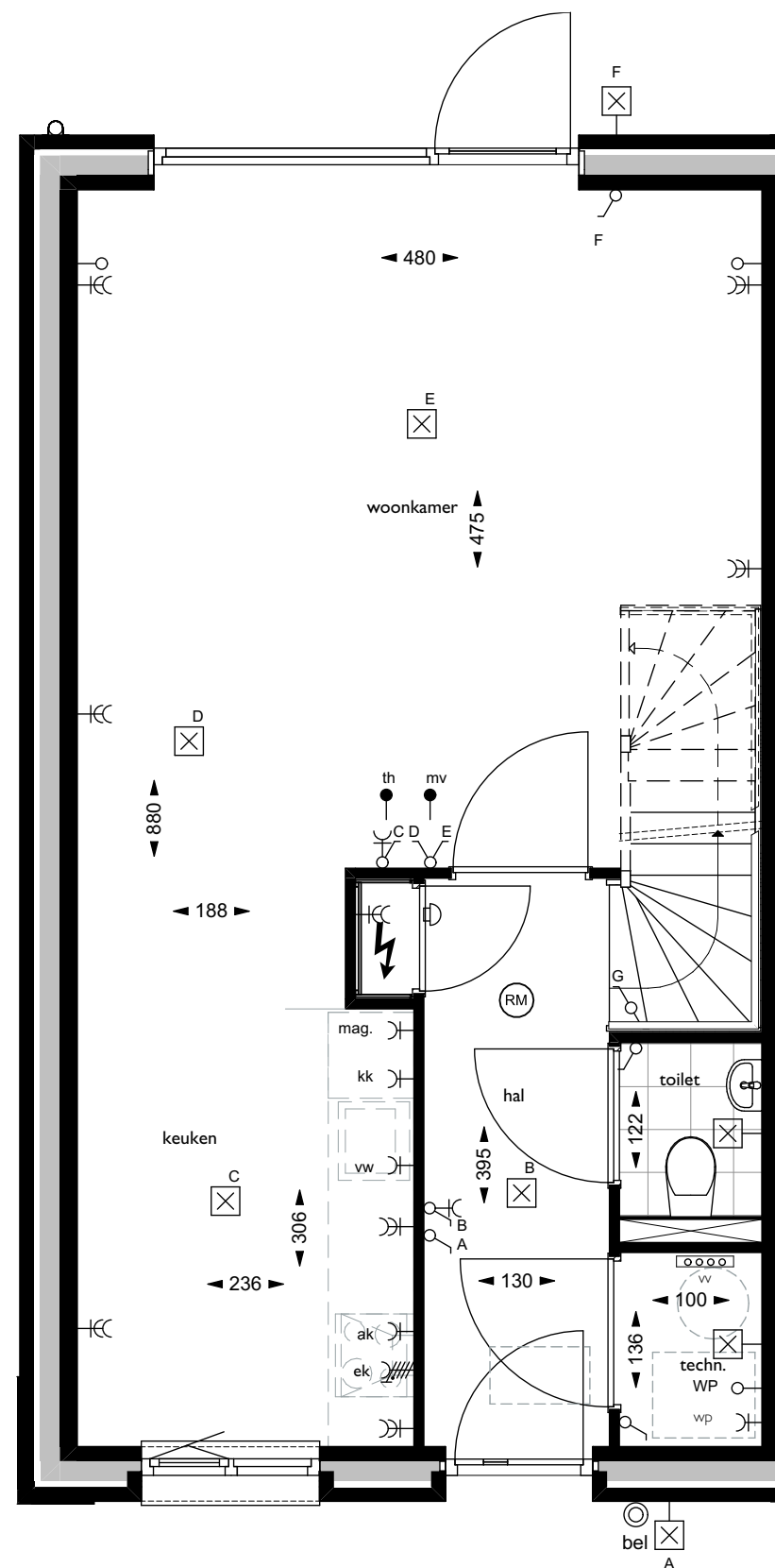
bouwnummer 43 begane grond
