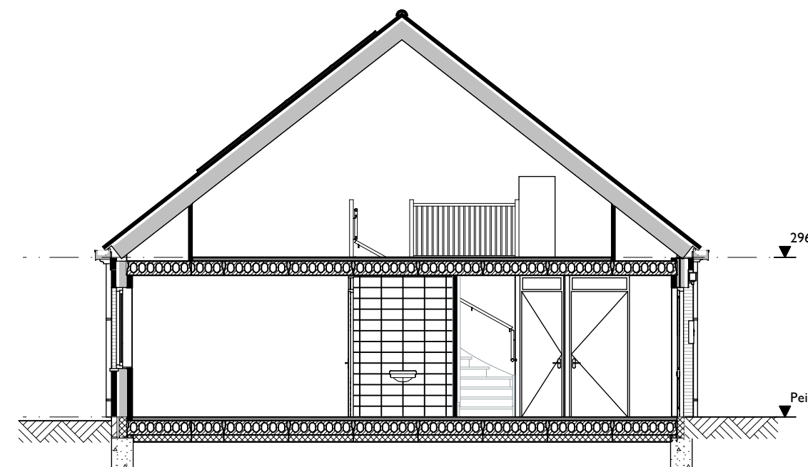
Doorsnede A-A
