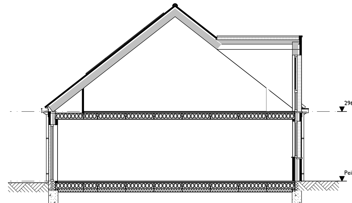
Doorsnede B-B
