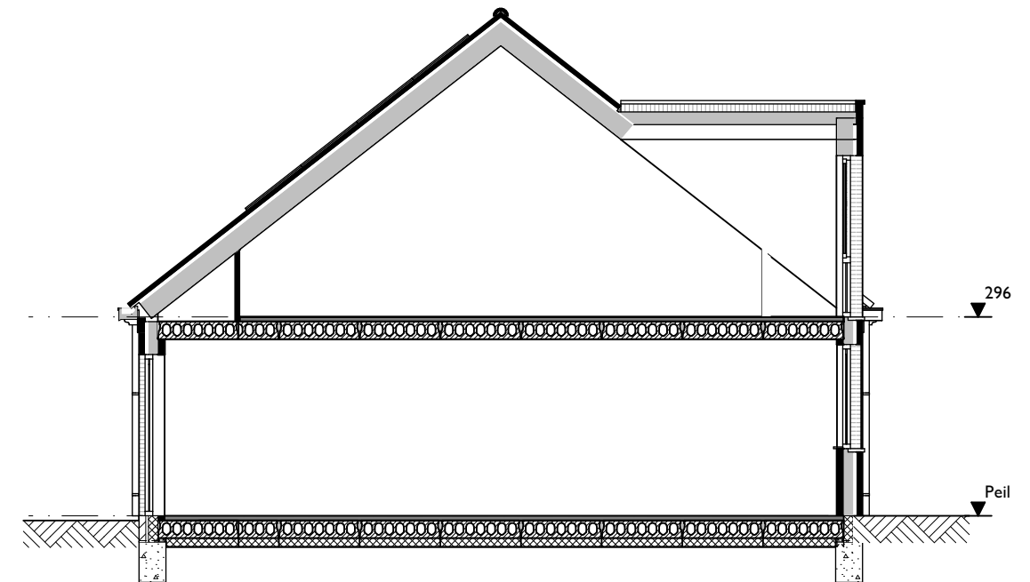
Doorsnede B-B
