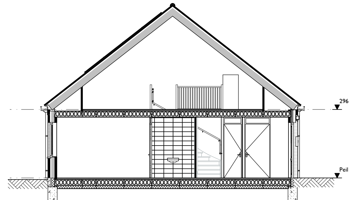
Doorsnede A-A
