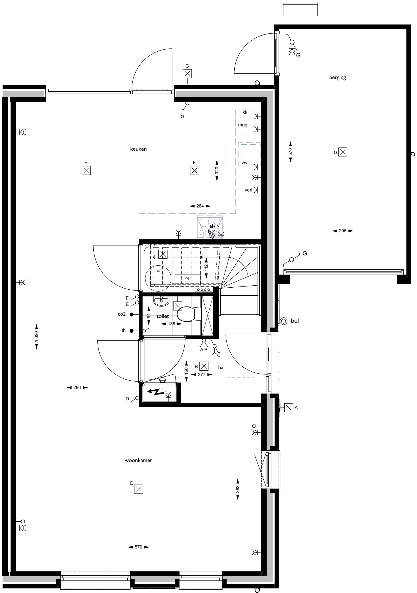
bouwnummer 74 begane grond
