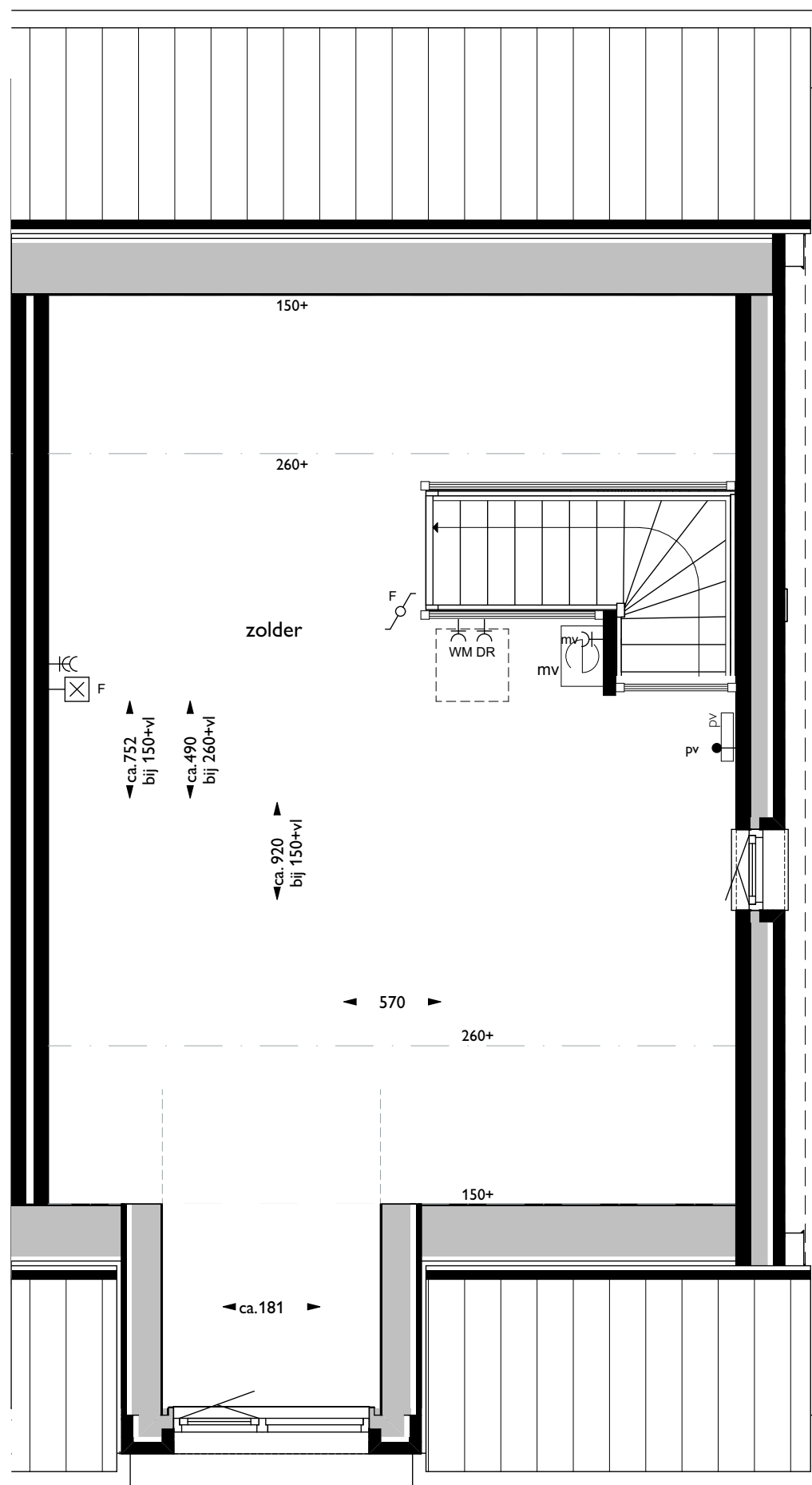
bouwnummer 74 tweede verdieping
