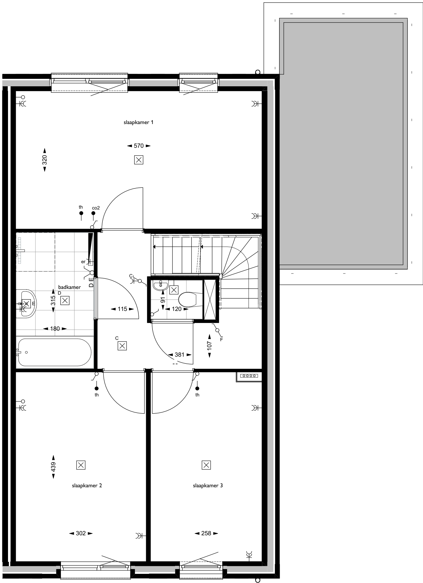
bouwnummer 74 eerste verdieping
