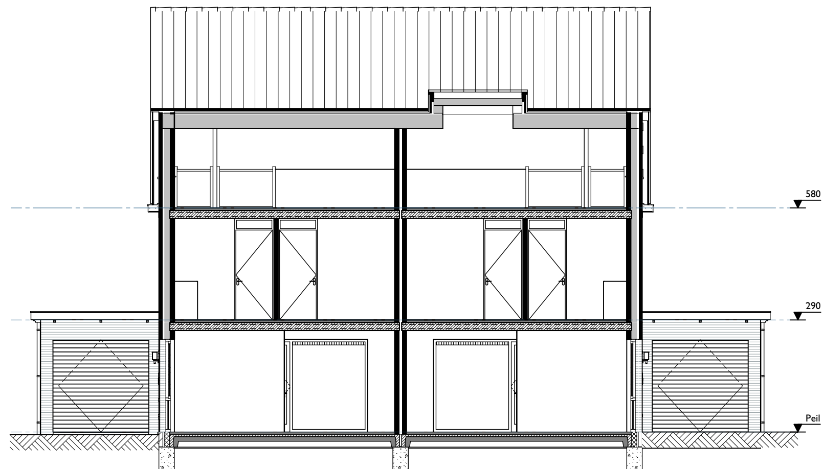
Doorsnede A-A
